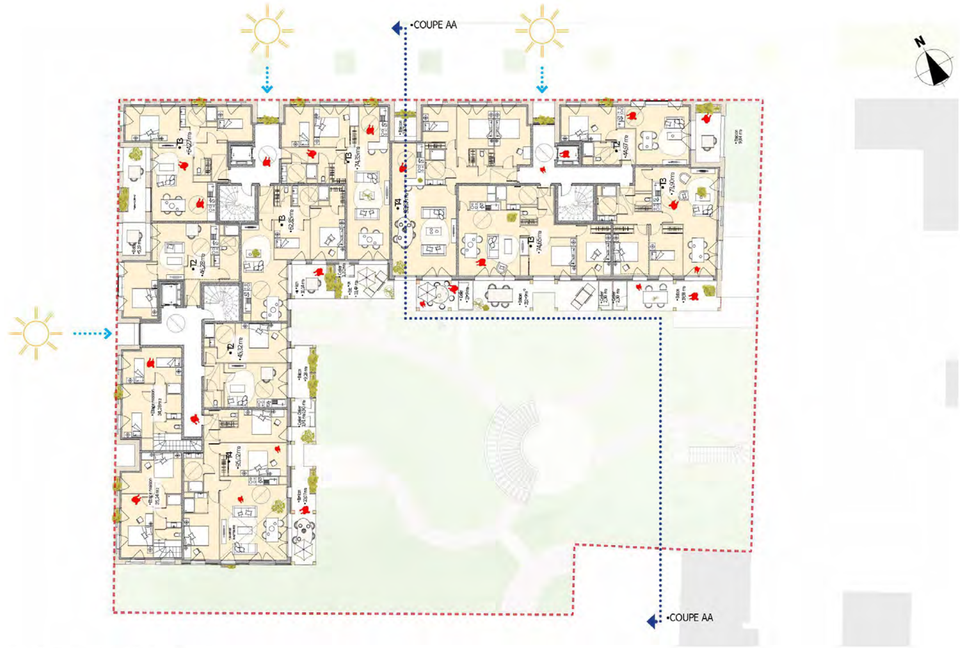
•PLAN DU PREMIER ETAGE 1/200
