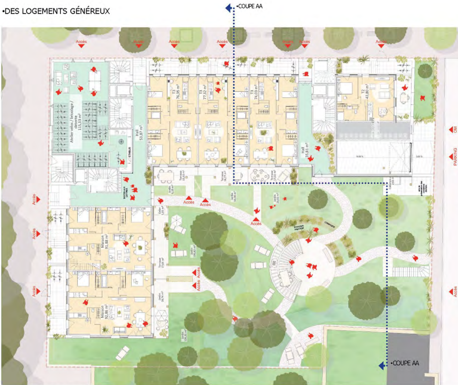
•PLAN DE REZ-DE-CHAUSSÉE 1/200
